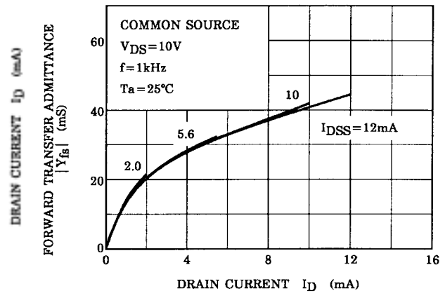
|Y_{fs}| - I_D
