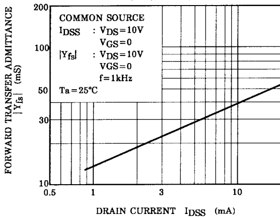
|Y_{fs}| - I_{DSS}
