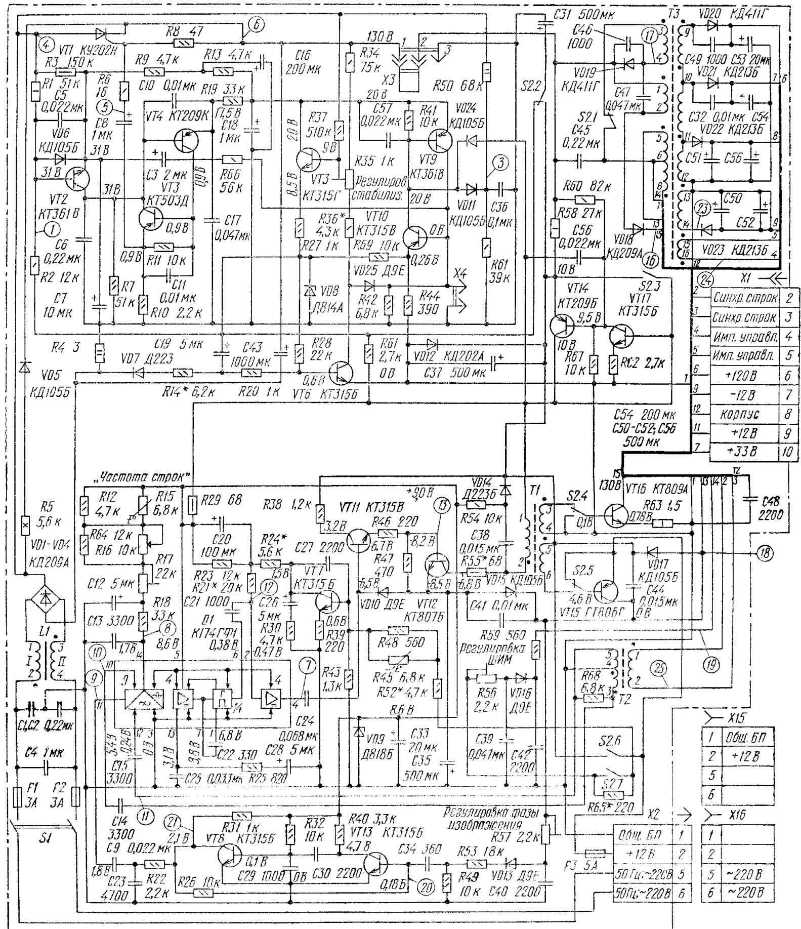
Принципиальная схема БП телевизора «Электроника Ц-430» (3-й вариант)
