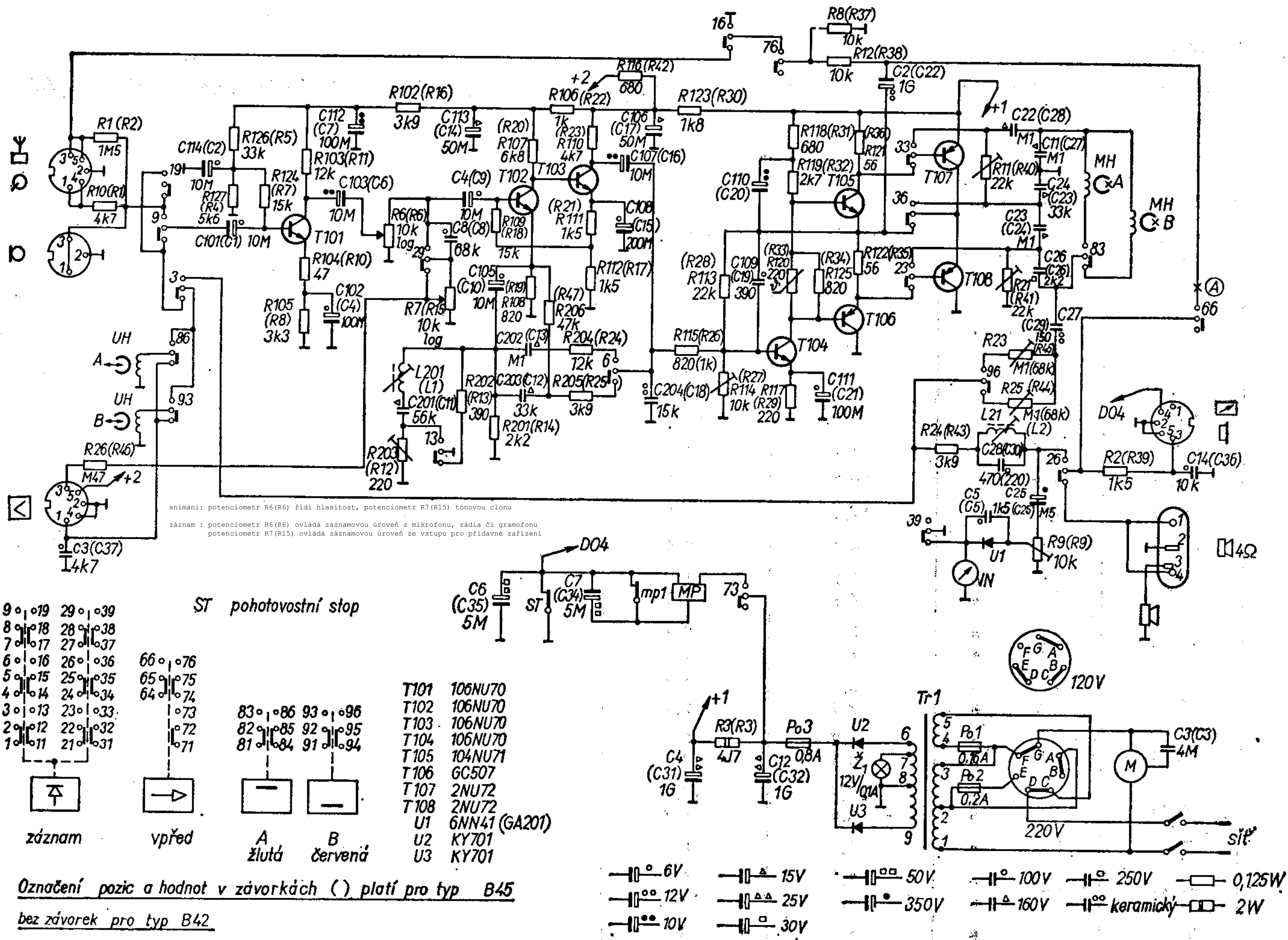
Obr. 107. Zapojení magnetofonů TESLA B 42 B 45
