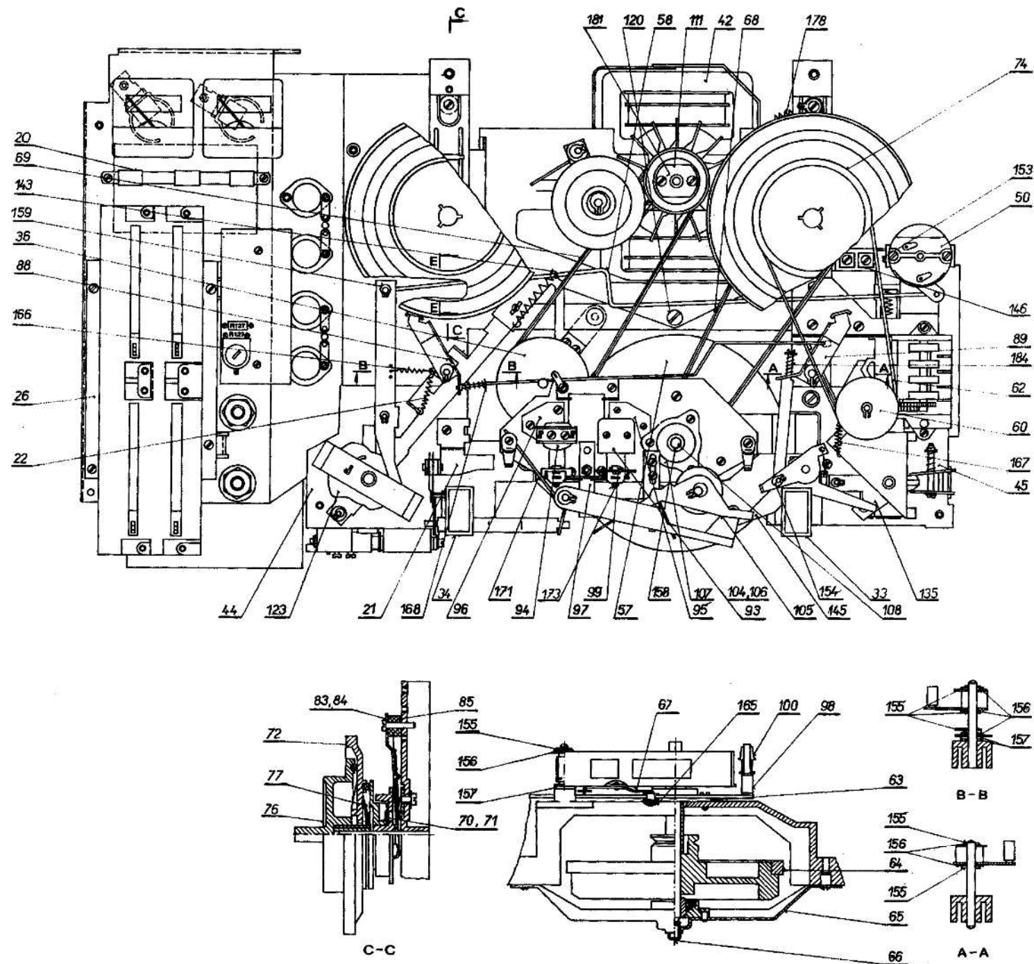
TESLA B100 / B100A / B101 - mechanická sestava
