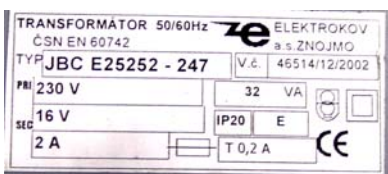
Štítek trafo
